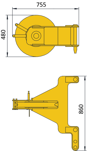
臂端单滑轮 83kg Single top 83kg
